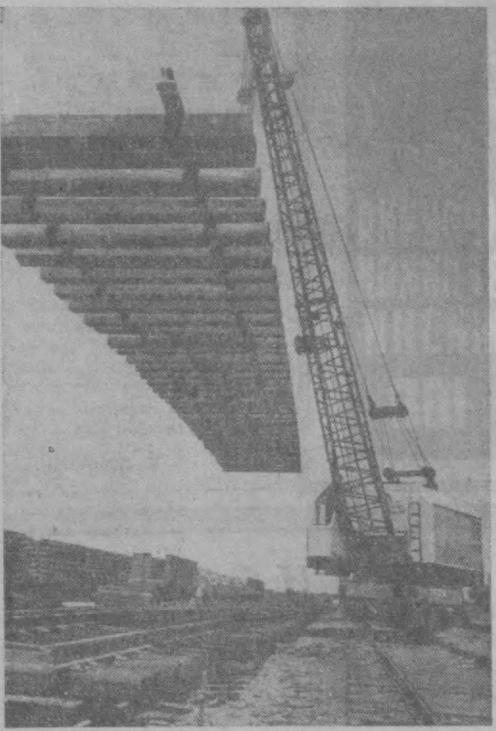
Завершена прокладка 126-километровой железнодорожной магистрали «Карши-Самарканд». На этом снимке вы видите Ушакладу последние рельсы, которую ведут рабочие строительномонтажного поезда № 313.
