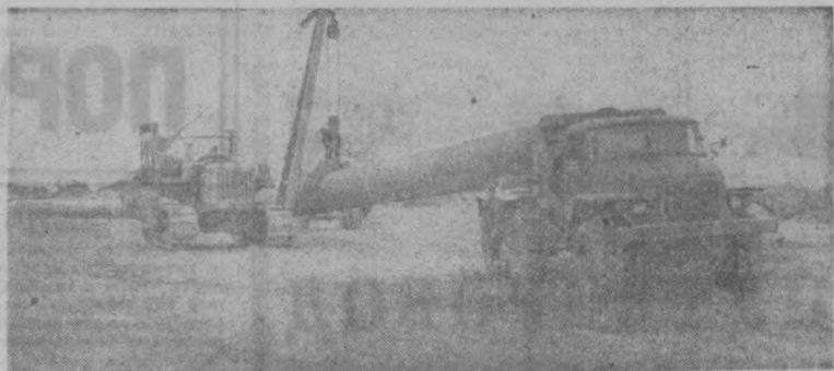
Успешно идет прокладка основного 487-километрового Транс-индийского магистрального газопровода, сооружаемого по инициативе советских специалистов. Осталось сварить несколько десятков километров труб. Впереди самый трудный участок — заболоченные рисовые поля Мазандерана. На снимке: погрузка плетей труб на участке 453-го километра вдоль берега Каспийского моря.
