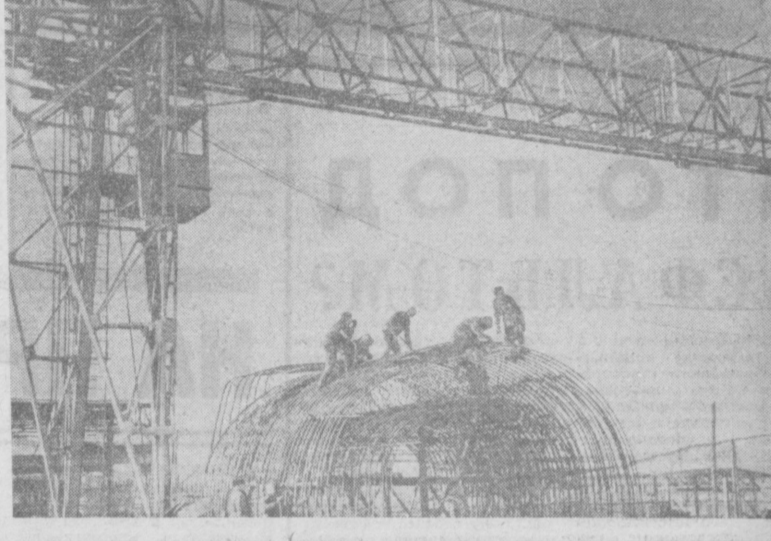
С большим напряжением трудятся строители Чарвакской ГЭС. Пожым ходом идут работы по облицовке бетоном опорных тоннельных водоводов. Монтажные управления специализированно устанавливают в тоннелях свыше 100 тонн арматурных каркасов. Сборка этих каркасов ведется одновременно на многих площадках. Затем их уже в готовом виде устанавливают в тоннелях. На снимке снимке вы видите сборку арматурных каркасов на одной из площадок стройки. А на снимке вверху — дипломированный сварщик управления спецработ Владимир Самолок — один из тех, кто вяжет эти металлические кружева. Владимир пришел на строительство Чарвакской ГЭС по комсомольской путевке в 1963 году и зарекомендовал себя отличным сварщиком. Сейчас со всем коллективом стройки он соревнуется за досрочное выполнение заданий пятилетки и за достойную встречу 100-летия со дня рождения В. И. Ленина. К этому времени агрегаты Чарвакской ГЭС должны быть в строю. Электричество Чарвака будет нести большую службу в промышленности, сельском хозяйстве, на транспорте. Пожым строители и о том, что их труд по достижению оценок трудящиеся в новой замечательной зоне отдыха.
