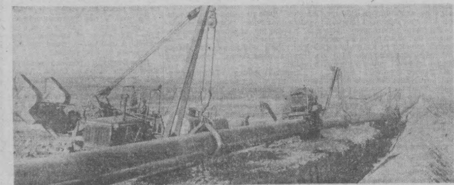
Более 200 километров труб уже уложили в траншеи строители крупнейшего в Средней Азии газопровода Мубарек — Ташкент — Фрунзе — Ала-Ата. Сейчас они подошли к отрогам Пуратинских гор. Этот трудный участок трассы газопровода будет штурмовать торпачи. Опыт работы в горах они приобрели во время строительства газопровода Джаржар — Ташкент. На снимке: идет укладка труб в траншею.
