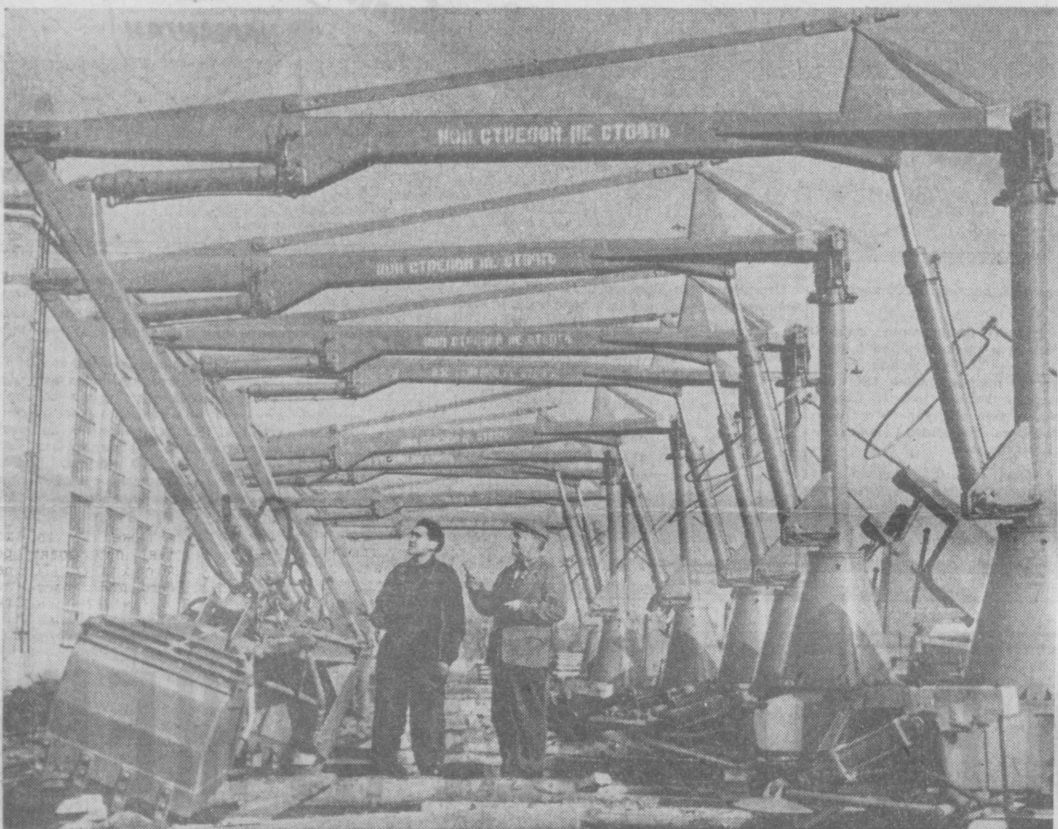
Широкое применение в народном хозяйстве нашли универсальные погрузчики марки «ПУ-0,5», выпускаемые Анджанским машиностроительным заводом. В нынешнем году коллектив предприятия наметил изготовить 1.200 таких механизмов. Все они сойдут с заводского конвейера досрочно, к 15 декабря. На снимке: контрольный мастер сборочного цеха М. Янушев и слесарь М. Чумарин проверяют партию готовых погрузчиков.
