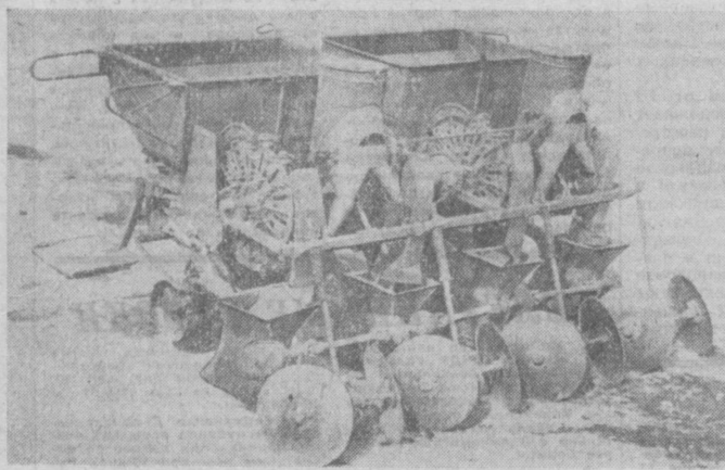
КАРТОФЕЛЕСАЖАЛКА ЧЕТЫРЕХРЯДНАЯ «СН-4Б».
