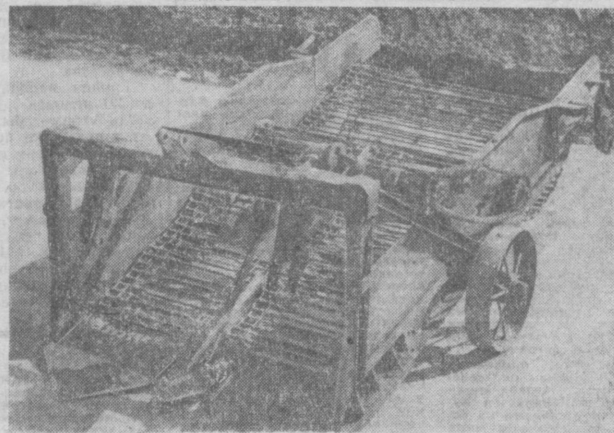
КАРТОФЕЛЕКОПАТЕЛЬ ДВУХРЯДНЫЙ «КТН-2Б».
