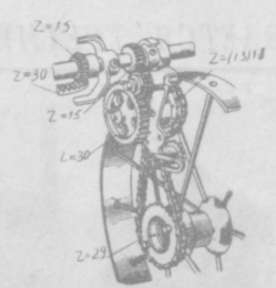
Рис. 2. Привод гнездующих аппаратов сеялки «СТХ-4Б».
