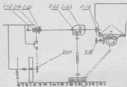
Рис. 3. Схема приводов высевальных и гнездующих аппаратов сеялки «СЧХ-4А-1».
