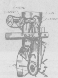
Рис. 1. Привод высевальных аппаратов сеялки «СТХ-4Б».
