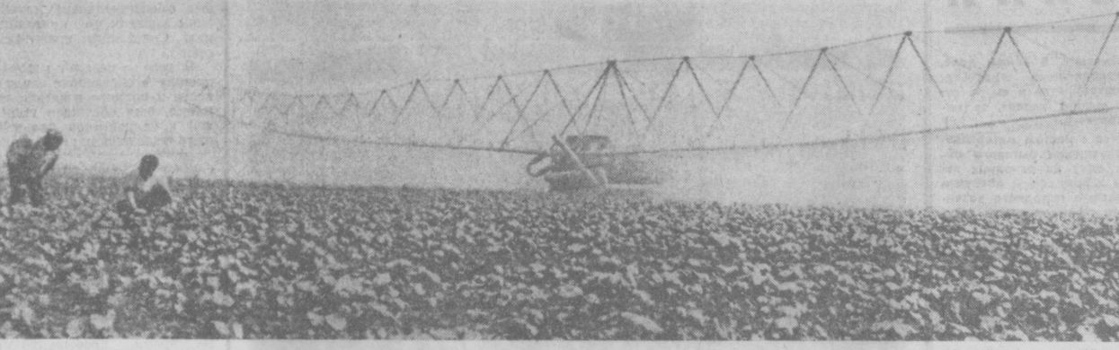
В ордене Ленина совхозе имени Пятилетия Узбекской ССР нынче впервые применят дождевальную агрегаты. Эффект беспорочный: одна машина заменяет десять поливальщиков, причем почва увлажняется равномерно.
