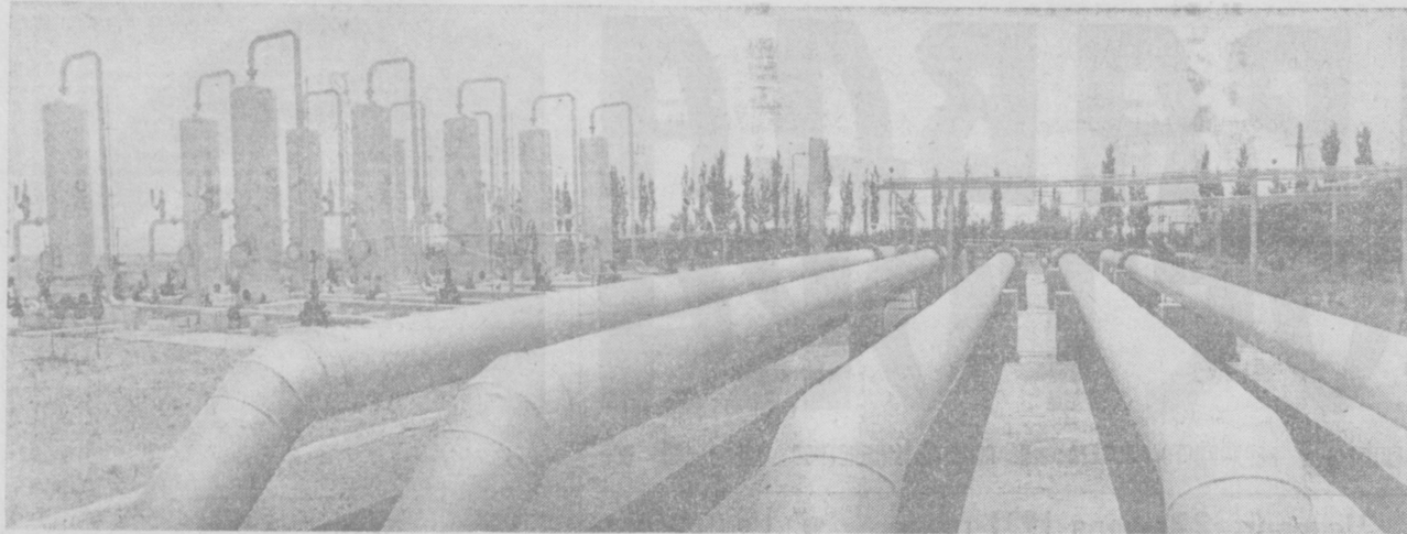
Газосборный пункт № 1 в Газли. Сюда со всех скважин собирается газ и здесь он готовится к дальней транспортировке на головное сооружение.
