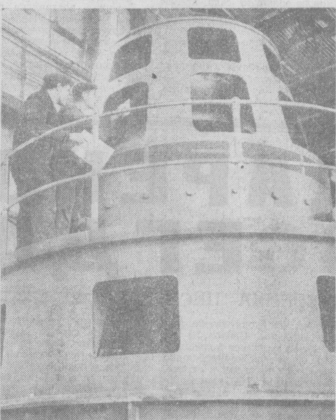
Монтажниками Чарвакской ГЭС досрочно смонтирована третья турбина. На снимке: монтаж агрегатов третьей турбины. Фото И. ГЛАУБЕРЗОНА и В. СИРОТКИНА.
