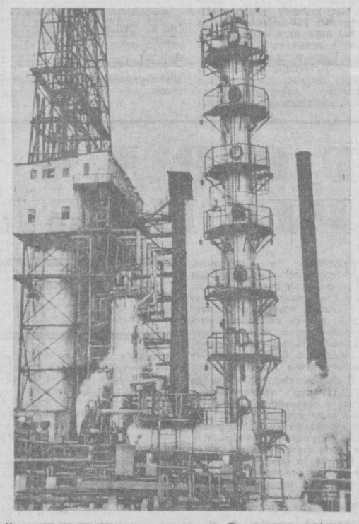
Конская технологическая установка Ферганского нефтеперерабатывающего завода. Фото В. СИРОТКИНА и И. ГЛАУБЕРЗОНА.
