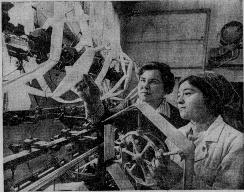
В одном из цехов Ташкентской опытной шелкоткацкой фабрики производится размотка нитонов, испытание шелковой пряжи. На снимке: контролер технического процесса Ф. И. Ахмедова (слева) и работница М. Базарбаева у мотальной машины. Фото И. ГЛАУБЕРЗОНА и В. СИРОТКИНА.
