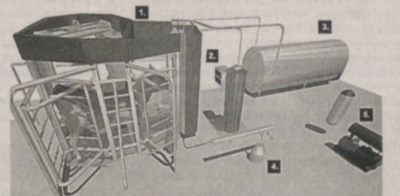
1 сигир соғиш кабиниси. 2 сут сифати текшириладиган тизим. 3 тайёр сут баки. 4 сифатсиз сут учун идиш. 5 сут сепаратори.
