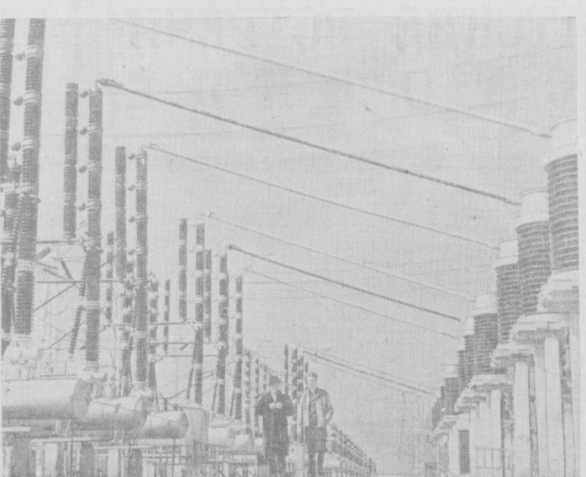
Проект Директив XXIII съезда КПСС по пятилетнему плану развития народного хозяйства предусмотрено завершение строительства Ташкентской ГРЭС — флагмана энергетики республики. Ее мощность будет доведена до одного миллиона девятиста тысяч киловатт. Четыре агрегата общей мощностью шестьсот тысяч киловатт, работающие на природном газе, уже встали под промышленную нагрузку. Значительно раньше срока завершено строительство открытой электроподстанции для будущей ГРЭС. Монтаж плато энероблока ведется с опережением установленного графика. На снимке: открытая электроподстанция ТашГРЭС.
