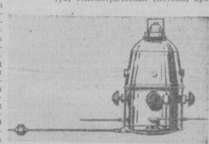
Автоматическая станция «Луна-10».
