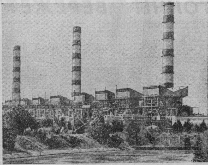
Общий вид Ташкентской ГРЭС. Фото И. ГЛАУВЕРЗОНА и В. СИРОТКИНА.
