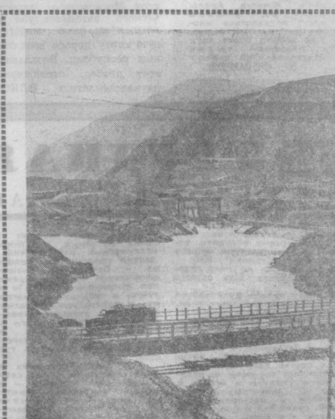
Чарванская ГЭС — всемирная стройка. Ее сооружают представители города семи национальностей. Свыше 600 предприятий страны поставляют Чарвану механизмы, машины, оборудование, материалы. На этом снимке вы видите отводной канал.
