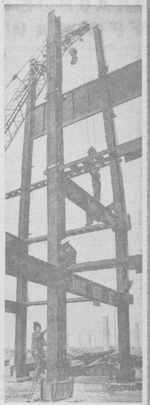
На снимке: монтаж металлических конструкций склада готовой продукции Алмалыкского химического завода. Фото А. ПАЛЕХОВА.
