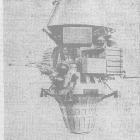
«Луна-12» автомат станцияси. 1. Астроориентация системаси микро органлари учун газ солинган баллонлар, 2. Фототелевизион курилма, 3. Иссиқликнинг тартибга солиш радиатори, 4. Радиометр, 5. Прибор қўйилмайдиган жой, 6. Кивий батарея, 7. Астроориентация системасининг оптик-механик бломи, 8. Антенна, 9. Астроориентация системасининг электрон бломи, 10. Бошқарувчи двигател, 11. Соловчи тормоз двигател устуқаси. ТАСС фотохроникаси.
