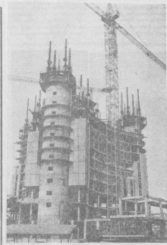
Все выше поднимаются конструкции строящейся в столице Узбекистана гостиницы «Москва». Монтажные строительные бригады в этот момент поднимают на очередную «шаг» перекрытия. Единственный метод подъема перекрытия позволяет на короткое время строить. Снаружи здание будет обложено керамзитобетонными панелями.
