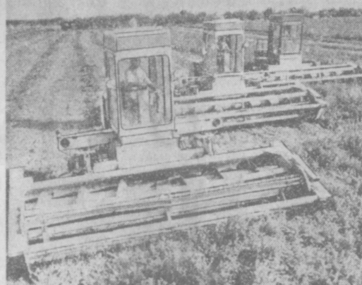
Сенокос в совхозе «Дабити» Ангаринского района. Два механизированных нормозаготовительных отряда ведут укос люцерны. Один из них укомплектован высокоскоростными комбайнами «Е-301» производства ГДР. Производительность одного такого комбайна в 10 раз выше «ИР-15». Механизаторы совхоза в этом году за 5 укосов обязались получить с каждого из 600 гектаров более 200 центнеров люцернового сена, что на 50 центнеров больше прошлогоднего.
