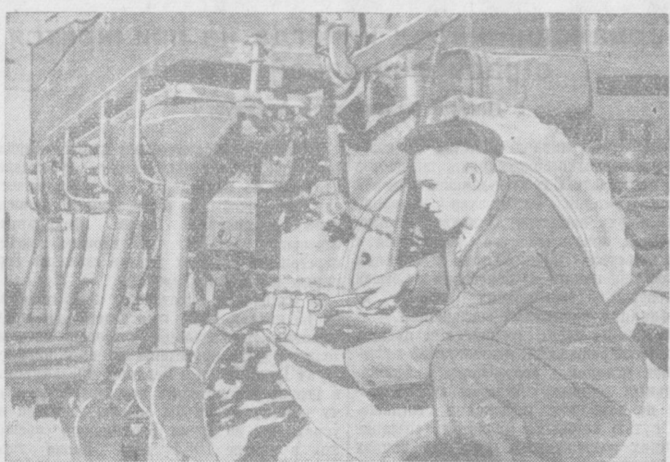
Механизаторы Дагбитской МТС Самаркандской области ведут работы по переделке пропашных тракторов, культиваторов, сенокос и другого сельскохозяйственного инвентаря для обработки хлопчатника на суженных междурядьях. На снимке: сесарь комсомолец П. С. Шелобаев. Работая на переделке СУЗ-а на ширину междурядий 45 см., он систематически перевыполняет норму выработки до 200 процентов.
