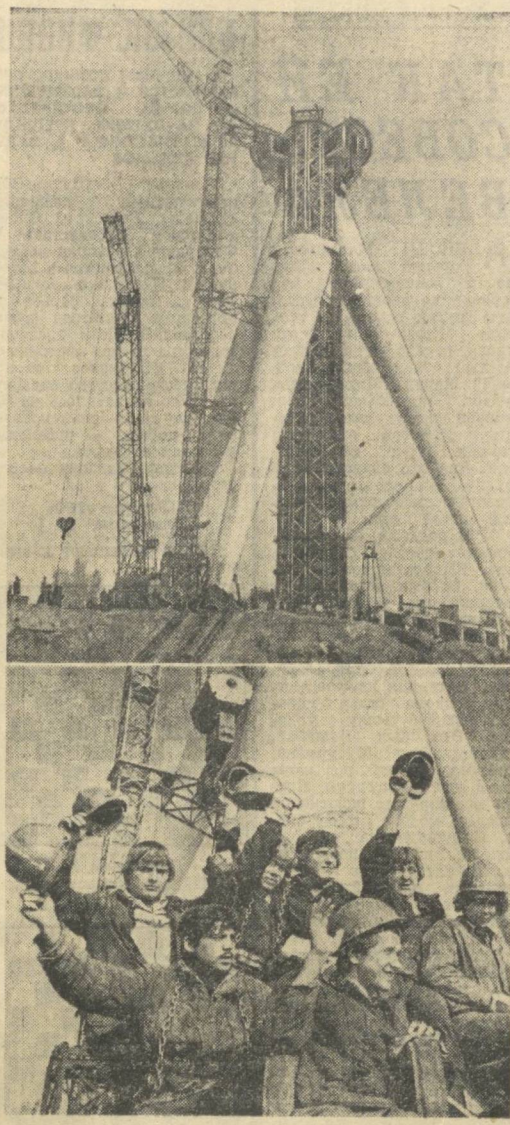
Успешно справились с подъемом третьей, последней из «ног» строящейся телебашни в Ташкенте коллектив Ленинградского монтажного управления № 26 треста «Спецстройинструкция». На снимках: сверху — так сейчас выглядит телебашня; внизу — они участвовали в подъеме третьего подкоса телебашни длиной 100 метров и весом 500 тонн.
