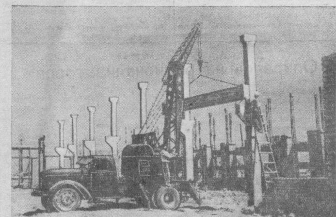
На снимке: монтаж механического цеха из железобетонных конструкций в третьей Беговатской МТС Ташкентской области. Фото А. Кима. (Фотохроника УзТАГ).
