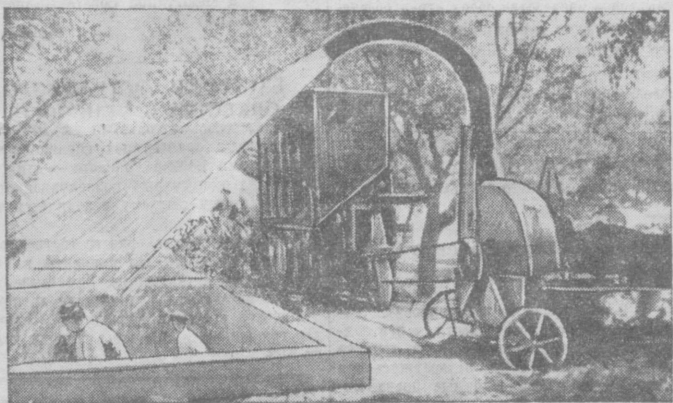
В колхозе имени Молотова, Чархинского района, для измельчения стеблей кукурузы на силос используют хлопкоуборочную машину. На снимке: общий вид агрегата, работающего на измельчении стеблей кукурузы на силос. Фото А. Кузьменко. (Фотохроника ТАТА).
