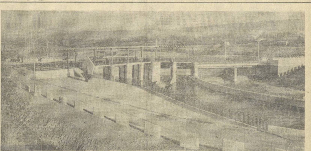
На реке Исфайрамской возле города Кувасай сдано в эксплуатацию мощное гидротехническое сооружение — Пальманский гидроузел. Ввод этого сооружения с автоматическим управлением поможет улучшить орошаемость более 30 тысяч гектаров хлопковых полей, виноградников и садов в Кувасайском, Ферганском, Ферганском районах, а также во Ферганском районе Киргизии. На снимке: верхний бьеф гидроузла. Фото Г. БОГНО, (УзТАГ).
