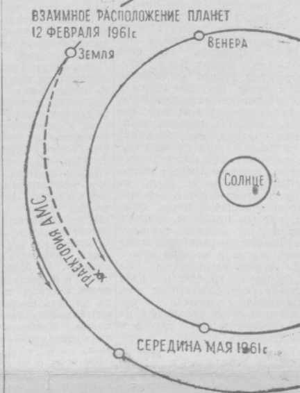
На схеме показан участок солнечной системы и взаимное расположение Земли и Венеры в момент старта автоматической межпланетной станции (АМС) и в момент ее востри с планетой-целью.
