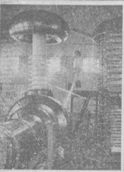
МОСКВА. В Институте атомной энергии имени И. В. Курчатова в течение 25 лет проводятся исследования с целью осуществления управляемой термоядерной реакции. Овладевая ею — значит одолеть человечество неиссякаемым источником энергии. На снимке: силовоточный ускоритель электронов «Ангара-1» для термоядерных исследований. Старший техник Г. М. Тихонов осматривает высокоскоростной ввод ускорителя.
