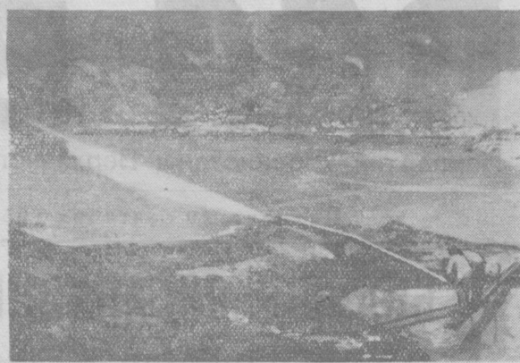
На Ангренском угольном разрезе широким фронтом производятся вскрышные работы при помощи гидромониторов. Мощные струи воды разрыхляют грунт, который по трубам уносится в отвальное русло. Этот способ намного ушелешает добычу угля. На снимке: гидромонитор за работой. Фото А. Огий.
