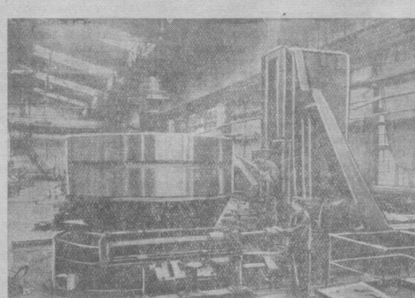
Ленинград, Кировский завод. На снимке: обработка колеса редуктора турбозубчатого агрегата в механическом цехе № 18. За работой зуборезы П. Н. Иванов (справа) и В. И. Михайлов. Они выполняют до двух норм за смену.
