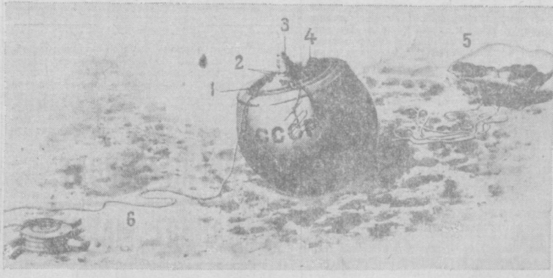
Венера юзасига қўйирилган «Венера-8» станциясининг туширилувчи аппарати. 1. Атмосфера ҳарорати ва босим датчиклари. 2. Ёрилиш ўлчам датчиги. 3. Асосий антенна. 4. Ташқарига чиқариладиган антенна (оттагунга қарар). 5. Парашют (оттагундан сўнг). 6. Ташқарига чиқариладиган антенна (оттагундан сўнг).
