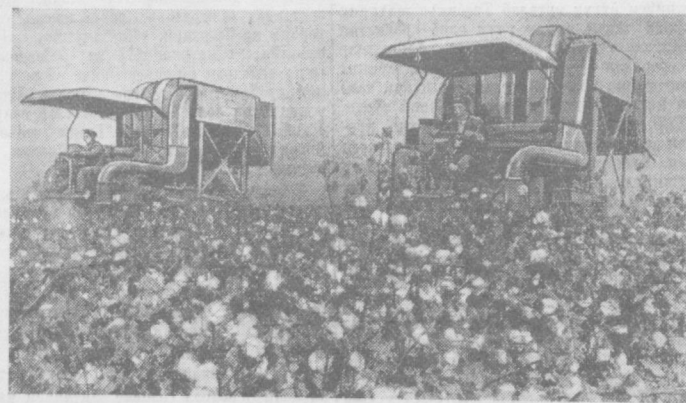
Суратда: илгор механик-ҳайдовчилардан Б. Узаиров ва Н. Киселев ўртоқлар Октябрь районидagi Киров номи колхозининг 1-ини бригадасида СХС—1,2 маркали янги машина блан пахта термоқдалар. И. Глауберзон ва В. Сироткин фотоси.
