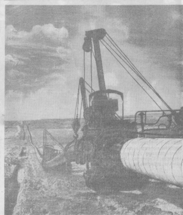
Ўзбекистон газ қардош Қозоғистон республикасининг қўпна саноат шаҳарларига ҳам етакчи берилади. Фото мухбири. А. Абальян олган бу суратда Оржоникидзе районидagi „Маданият“ колхозини территориясида Ўзбекистонга борадиган газ қувури ётқизиш ишлари ас эттирилган.
