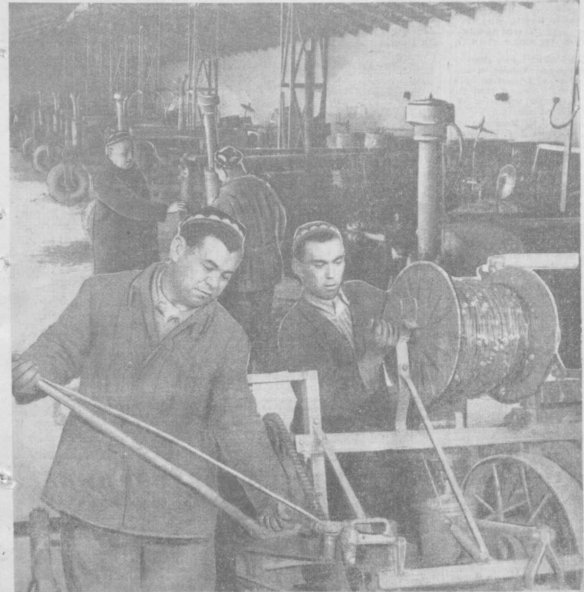
Оржоникидзе районидида «Маданият» колхозида техника экишга тахт қилиб қўйилди. Квадрат-улаб чигит экатиган етти ағ регат, айниқса, сифатли ремонтдан чиқарилади. Суратда: (олдинги қаторда чапдан) бригадда механикнинг ёрдамчиси И. Иноғомов ва тракторчи Х. Соляев ўртоқлар янги СХТВ-4 селласини регулировка қилмоқдалар.
