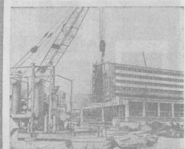
Германия Демократик Республикасида саноати йил сайини ривожлантириш чўққилар сари илдам бормоқда. Шу йилнинг дастлабки уч ойида ўтган йилгагина қисбатан саноат қурилиши 8 процентга ошди. Суратда: Йена — Зюд иссиқлик электростанциясининг қурилиши. Бу электростанция йил бариб этилаётган Лобе-ду шаҳрини электр қуввати билан таъминлайди.
