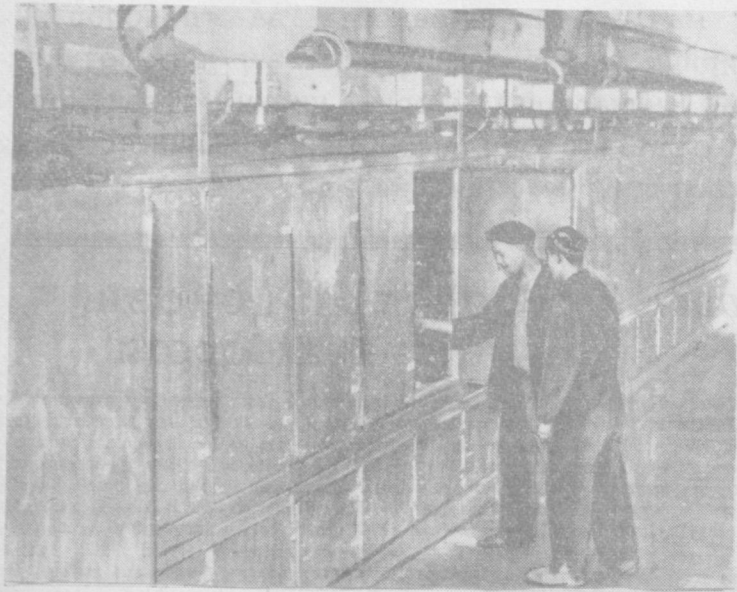
Суратларда: 1. электрод пехиди куритиб-тоблаш установ- насининг умумий кўриниши. 2. Контролер В. А. Бездуб ва пех бошлиги Г. А. Федулов тайёр маҳсулотлар сифатини кўздан кечирмоқдалар.
